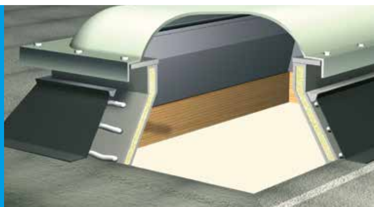
Exemple d'utilisation: tôles colaminées Wolfin au niveau du raccord de la coupole
